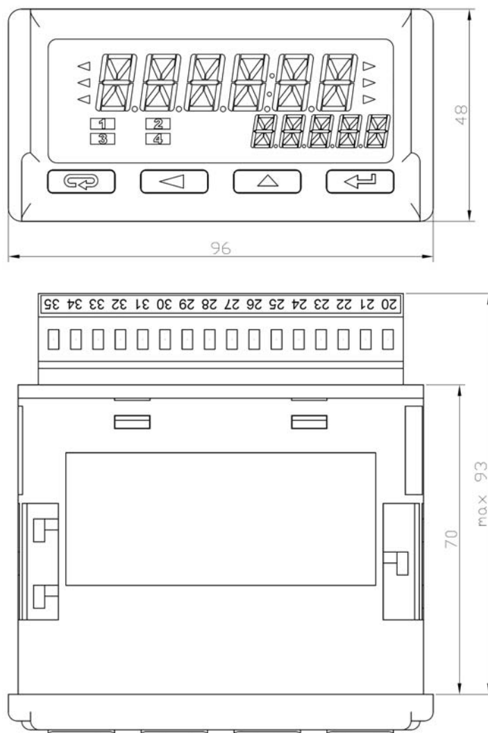
Rys. 3: Gabaryty miernika.
