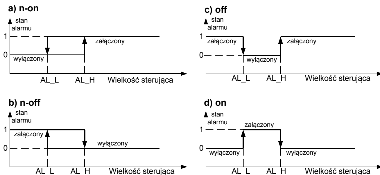
Rys. 11: Typy alarmów: a) n-on; b) n-off; c) off; d) on.
