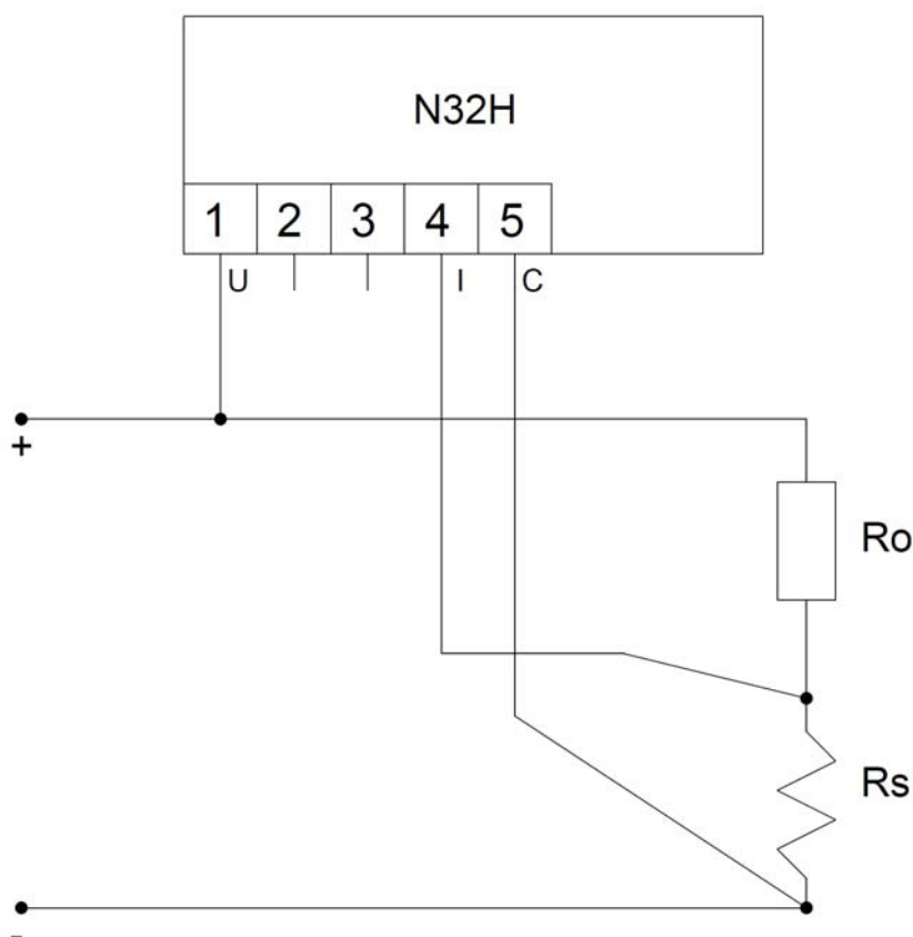
Rys. 6: Sposób podłączenia miernika N32H,
