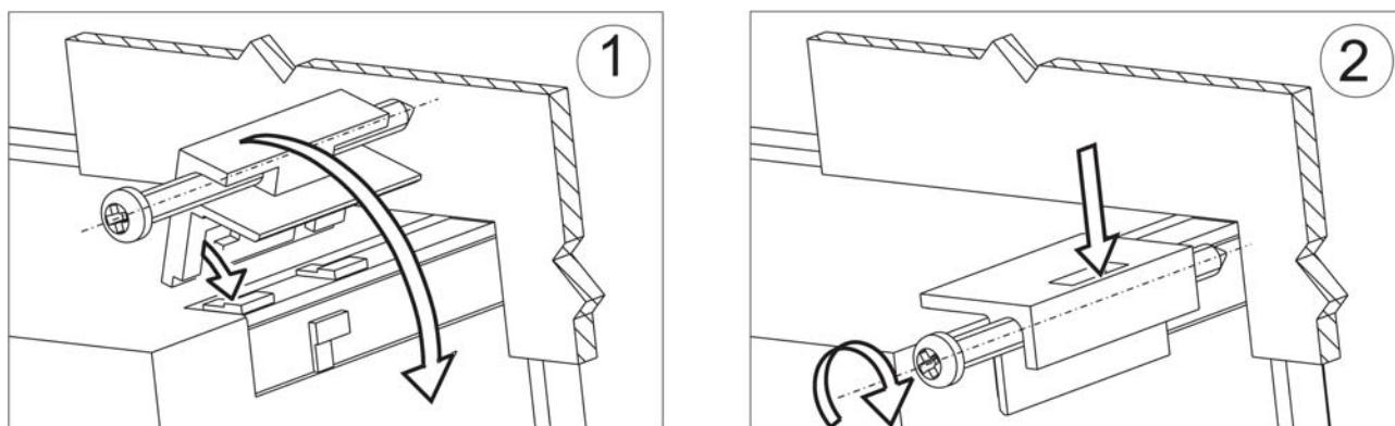
Rys. 2: Mocowanie miernika.
