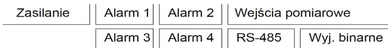
Rys. 4: Separacja galwaniczna w mierniku N32H.
